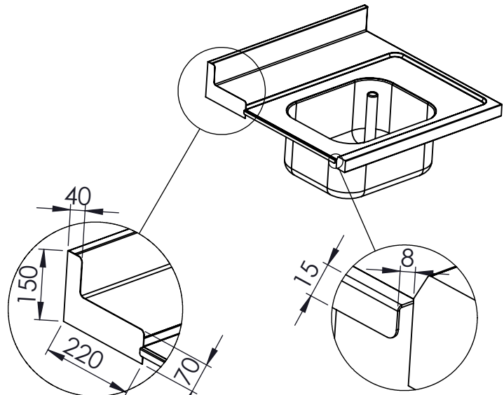
DETTAGLIO SCALA 1 : 10
