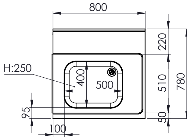
DETTAGLIO SCALA 1 : 10
